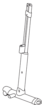
② 오른쪽 다리 x1 Right foot tube set x 1
